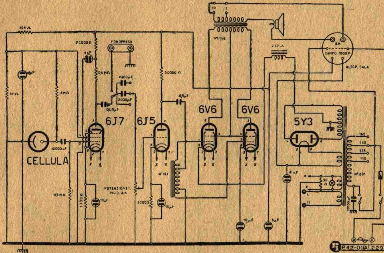
Lo schema elettrico dell'amplificatore Prevost mod. "121,, II Serie.
